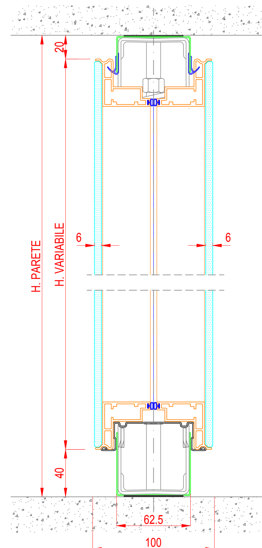
LUCE DOPPIO VETRO TEMPERATO SEZIONE VERTICALE
